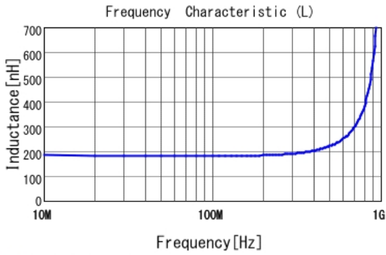
■ LQP03HQR18H02 L
