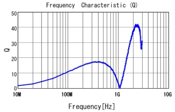
■ LQP03HQR18H02 Q
