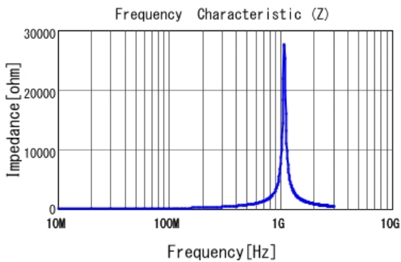
■ LQP03HQR18H02 |Z|
