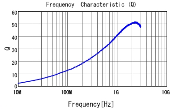
■ LQP03HQ9N1H02 Q
