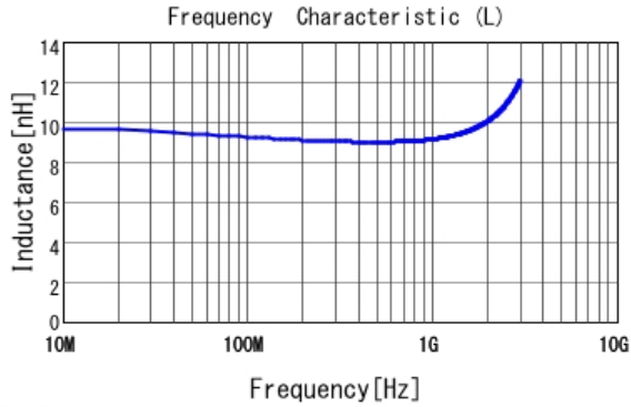
■ LQP03HQ9N1H02 L
