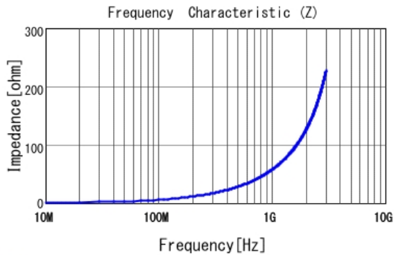
■ LQP03HQ9N1H02 |Z|
