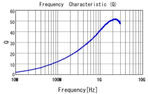
■ LQP03HQ8N2H02 Q
