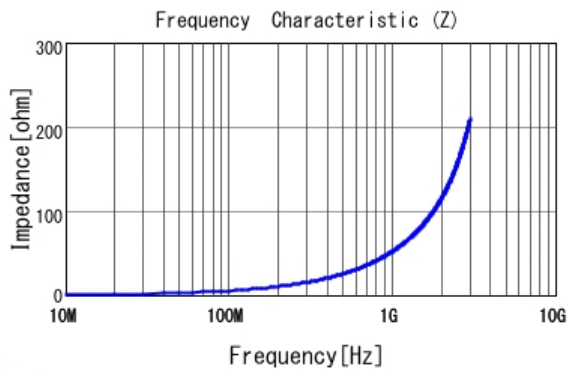
■ LQP03HQ8N2H02 |Z|
