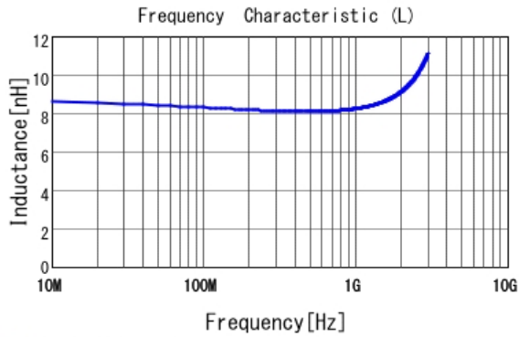
■ LQP03HQ8N2H02 L
