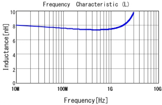
■ LQP03HQ7N5H02 L
