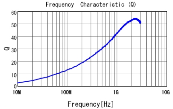
■ LQP03HQ7N5H02 Q
