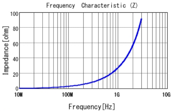
■ LQP03HQ4N3H02 |Z|
