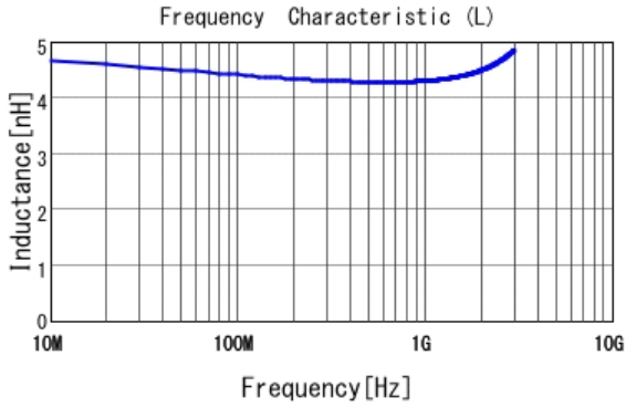
■ LQP03HQ4N3H02 L
