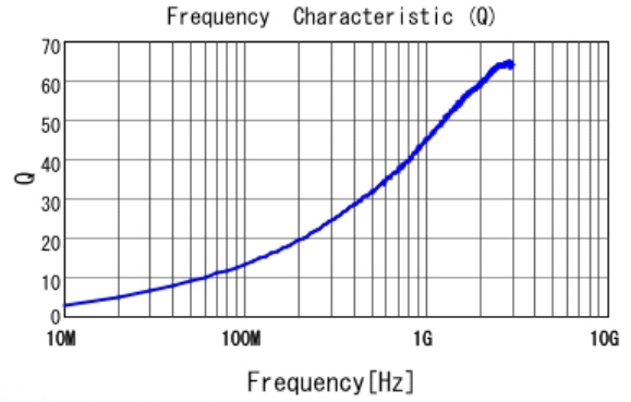
■ LQP03HQ4N3H02 Q
