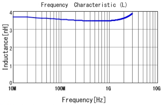
■ LQP03HQ3N5B02 L
