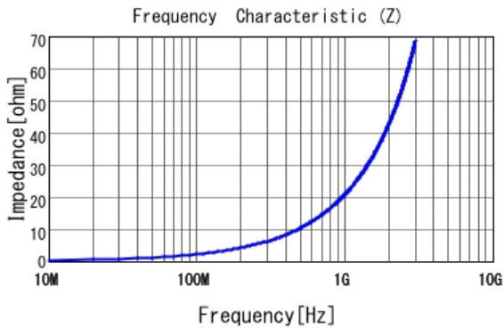
■ LQP03HQ3N3B02 |Z|
