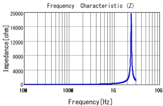
■ LQP03HQ39NH02 |Z|
