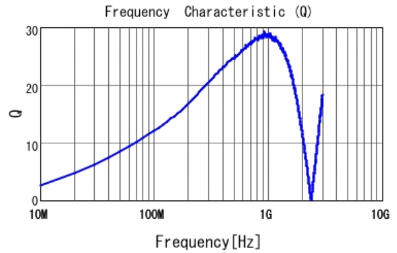
■ LQP03HQ39NH02 Q
