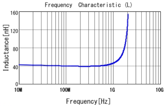
■ LQP03HQ39NH02 L
