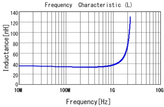
■ LQP03HQ33NH02 L
