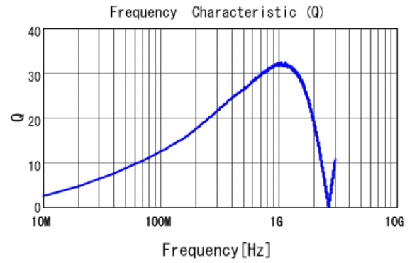
■ LQP03HQ33NH02 Q
