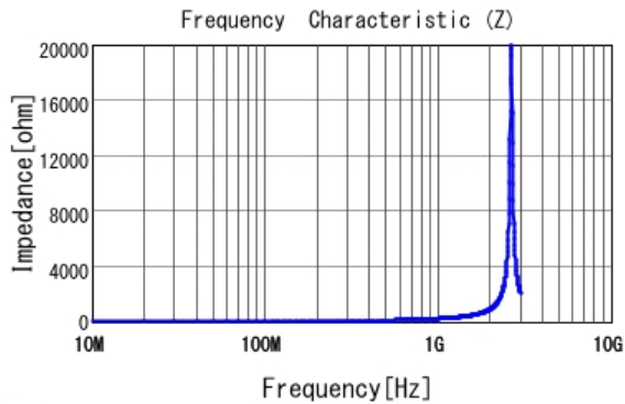
■ LQP03HQ33NH02 |Z|
