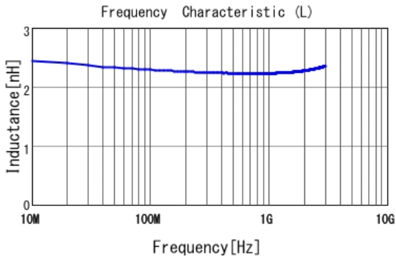
■ LQP03HQ2N2B02 L
