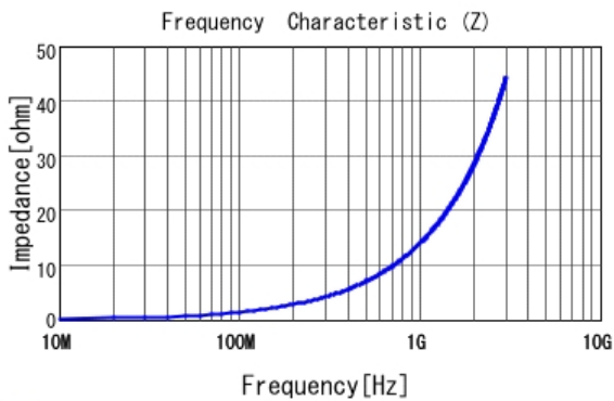
■ LQP03HQ2N2B02 |Z|
