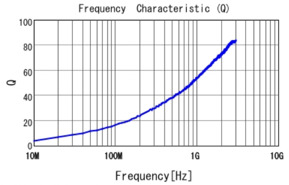
■ LQP03HQ2N2B02 Q
