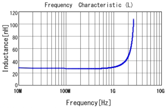
■ LQP03HQ27NH02 L
