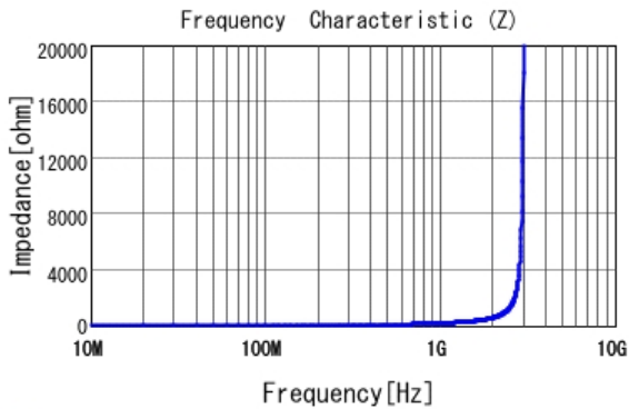
■ LQP03HQ27NH02 |Z|
