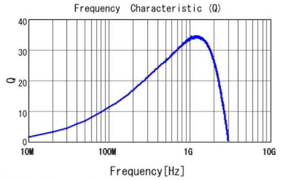
■ LQP03HQ27NH02 Q
