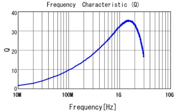
■ LQP03HQ22NH02 Q
