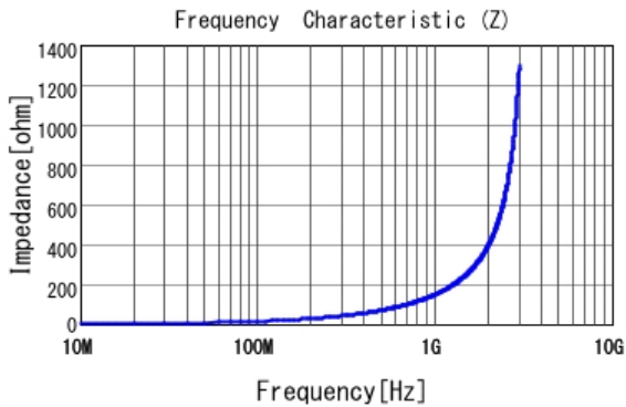
■ LQP03HQ22NH02 |Z|
