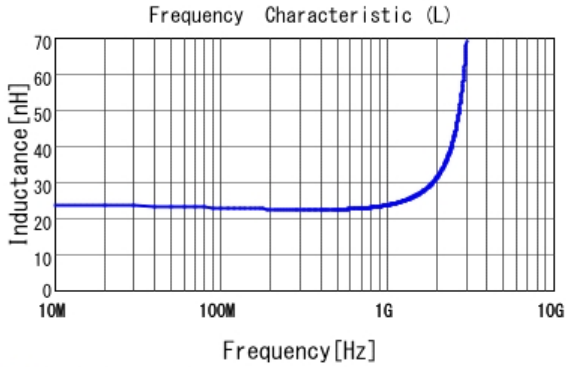
■ LQP03HQ22NH02 L
