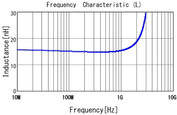
■ LQP03HQ15NH02 L
