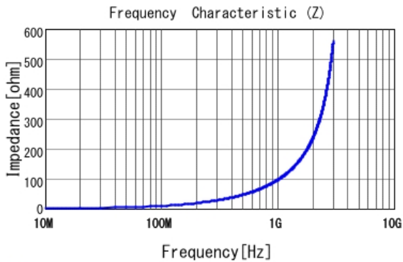
■ LQP03HQ15NH02 |Z|
