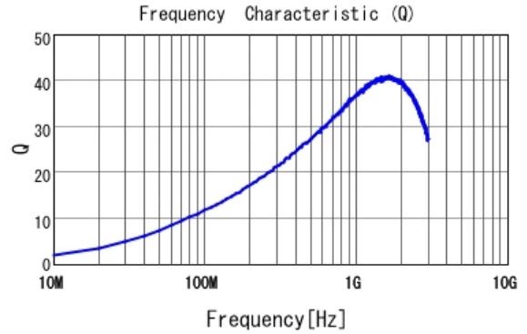
■ LQP03HQ15NH02 Q
