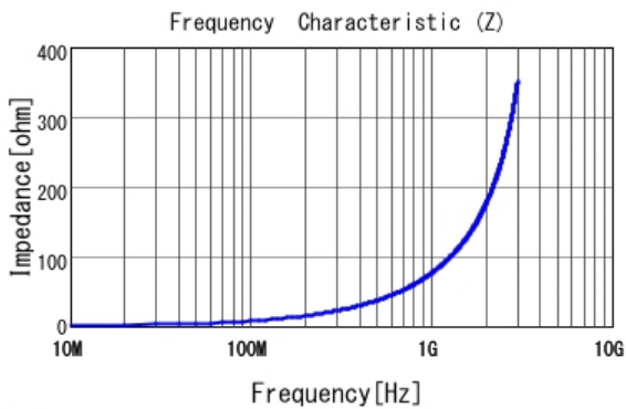
■ LQP03HQ12NJ02 |Z|
