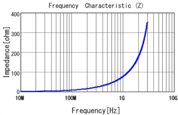
■ LQP03HQ12NH02 |Z|
