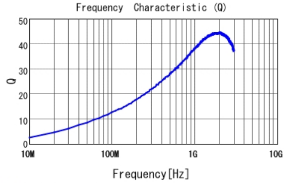
■ LQP03HQ12NH02 Q
