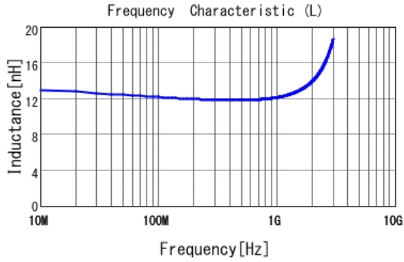
■ LQP03HQ12NH02 L
