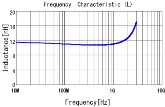
■ LQP03HQ11NH02 L
