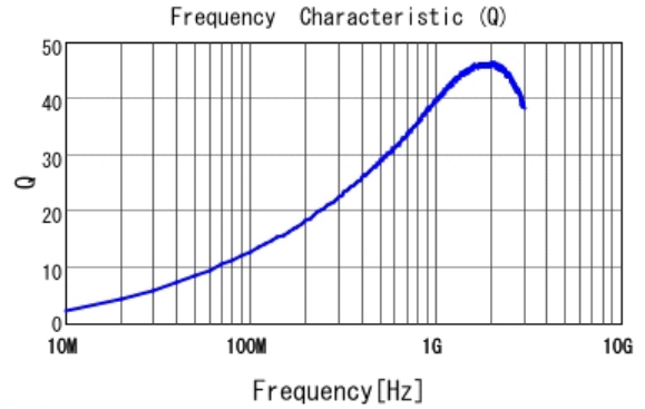
■ LQP03HQ11NH02 Q
