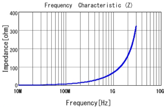
■ LQP03HQ11NH02 |Z|
