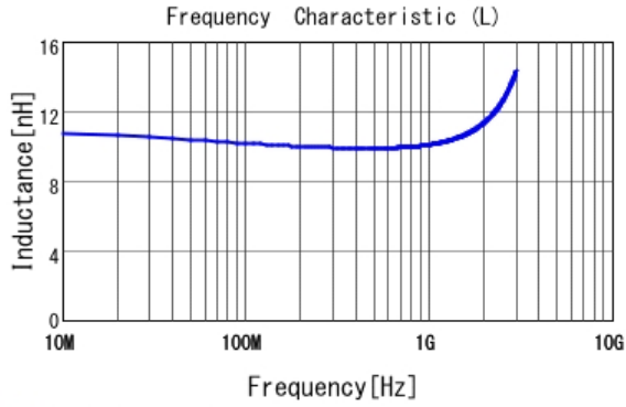
■ LQP03HQ10NH02 L
