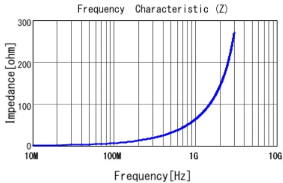
■ LQP03HQ10NH02 |Z|
