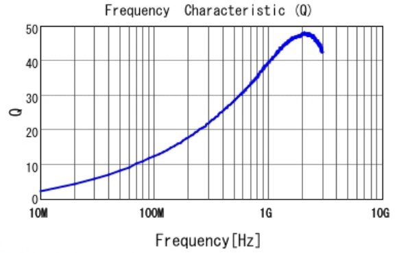
■ LQP03HQ10NH02 Q
