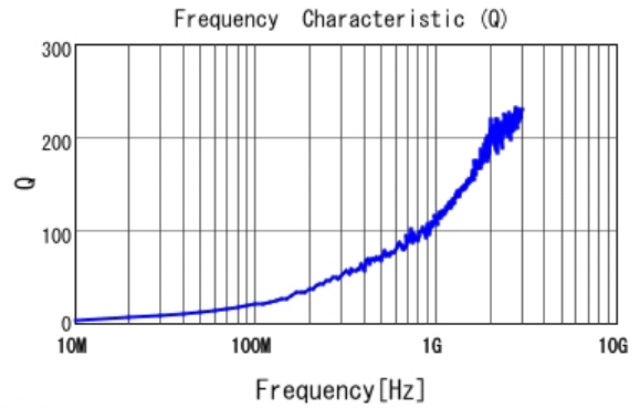
■ LQP03HQ0N8B02 Q
