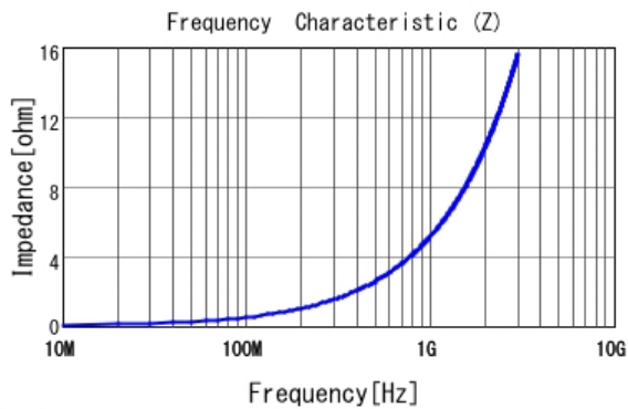
■ LQP03HQ0N8B02 |Z|
