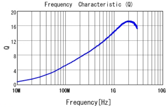
■ LQP02TQ18NH02 Q
