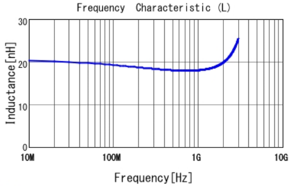
■ LQP02TQ18NH02 L
