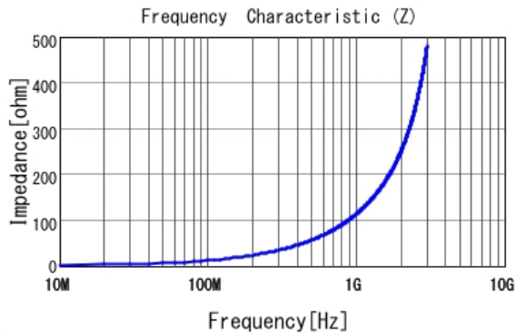
■ LQP02TQ18NH02 |Z|
