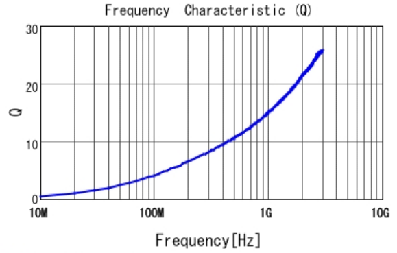
■ LQP02TN4N7H02 Q
