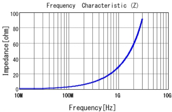
■ LQP02TN4N7H02 |Z|
