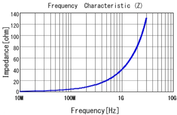
■ LQP02HQ6N2H02 |Z|
