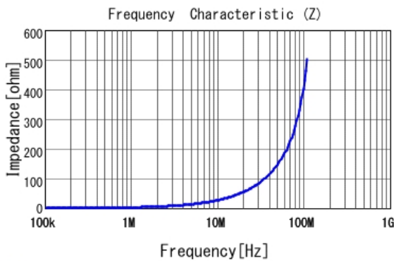
■ LQM2MPZR47NG0 |Z|
