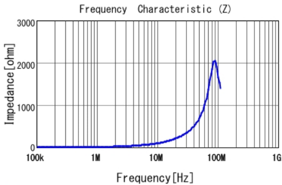
■ LQM2MPN1R5MG0 |Z|
