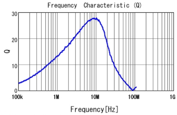
■ LQM2MPN1R0MEH Q
