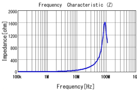
■ LQM2MPN1R0MEH |Z|
