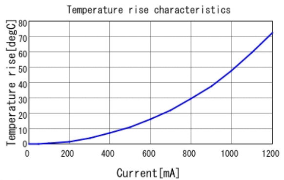
■ LQM21PN4R7MGS Temp. rise
