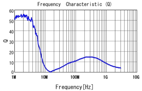
■ LQM21DN470M70 Q
