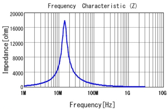
■ LQM21DN470M70 |Z|
