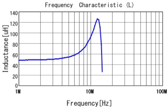
■ LQM21DN470M70 L
