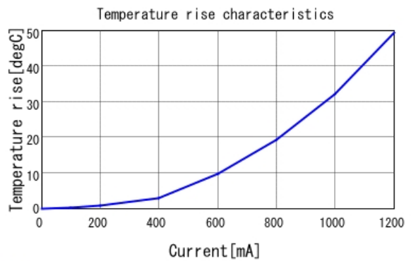
■ LQM18PZ2R2MCH Temp. rise
