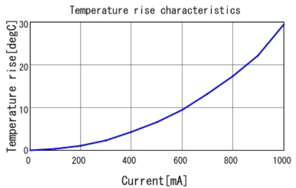
■ LQM18PNR47NC0 Temp. rise
