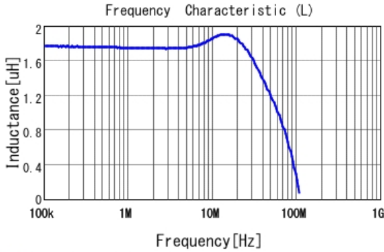
■ LQM18PN1R8NC0 L
