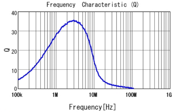
■ LQM18PN1R8NC0 Q
