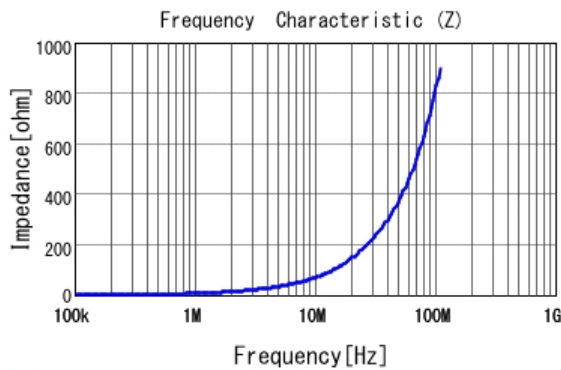
■ LQM18PN1R0MFH |Z|
