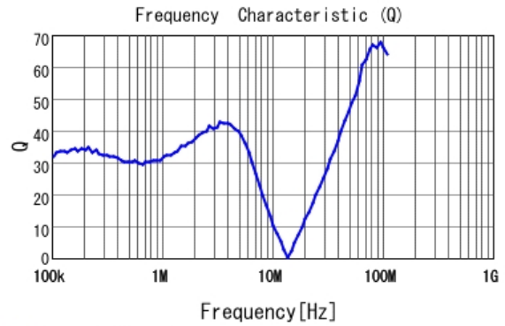
■ LQH5BPN220M38 Q
