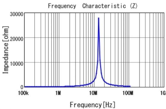
■ LQH5BPN220M38 |Z|
