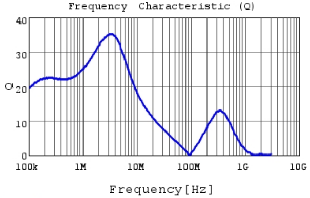
LQH5BPN1R5NT0 Q
