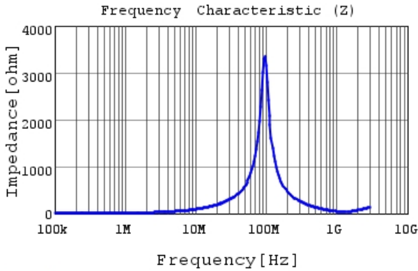
LQH5BPN1R5NT0 |Z|
