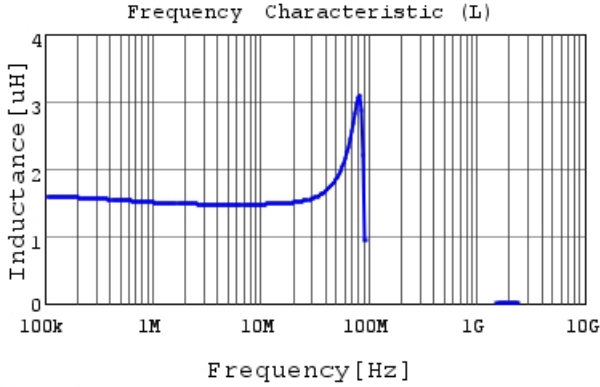
LQH5BPN1R5NT0 L
