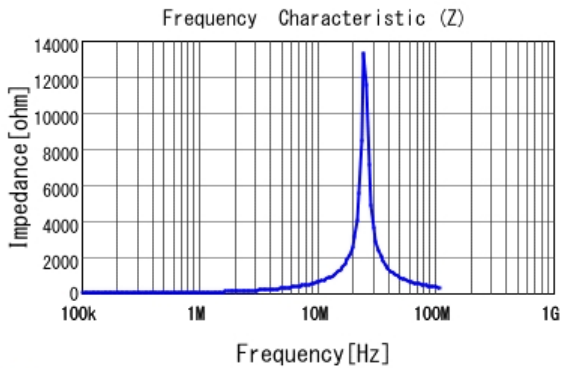
■ LQH5BPN100M38 |Z|
