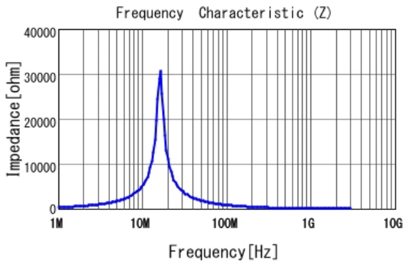
■ LQH3NPZ470MJR |Z|
