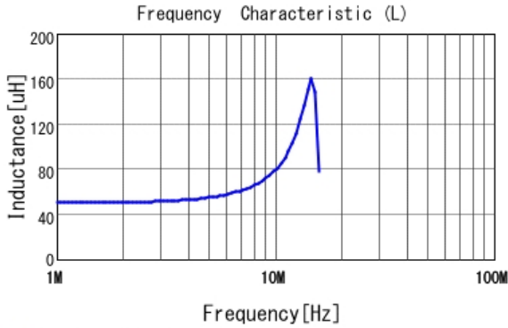
■ LQH3NPZ470MJR L
