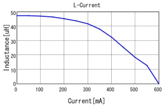
■ LQH3NPZ470MJR L-Current 20degC
