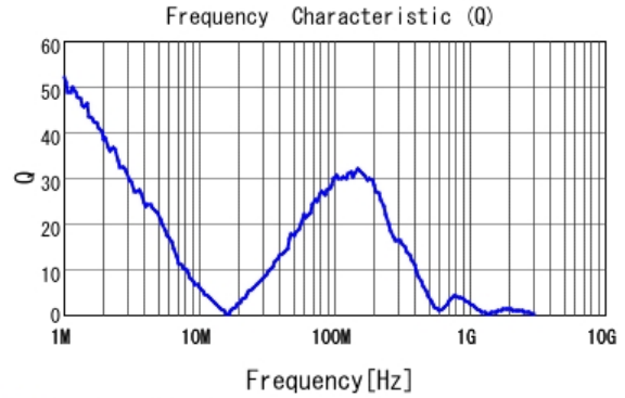
■ LQH3NPZ470MJR Q
