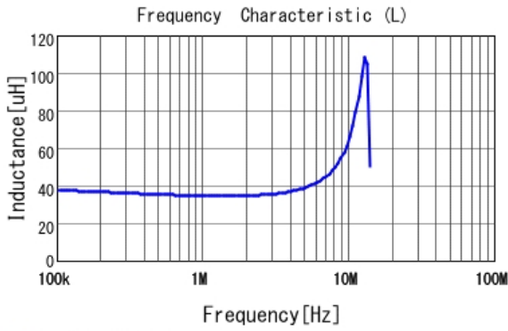
■ LQH3NPZ330MGR L
