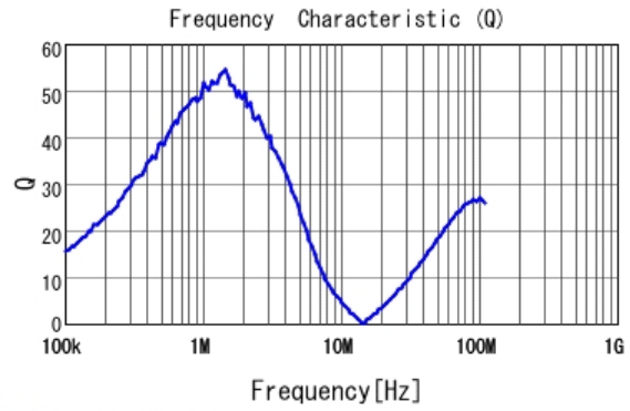
■ LQH3NPZ330MGR Q
