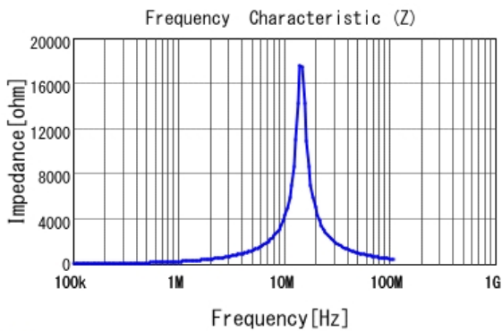
■ LQH3NPZ330MGR |Z|
