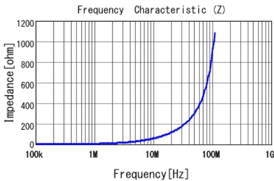
■ LQH3NPZ1R0MME |Z|
