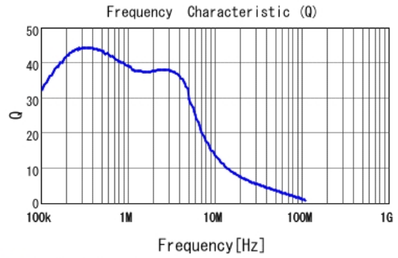
■ LQH3NPZ1R0MME Q
