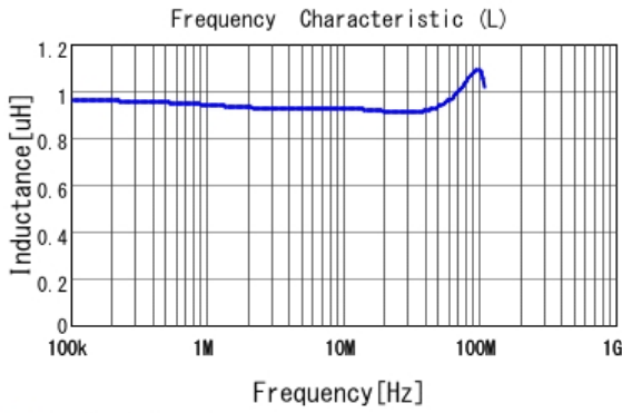
■ LQH3NPZ1R0MME L
