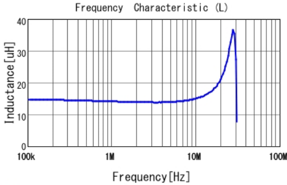
■ LQH3NPZ150MME L
