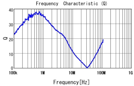
■ LQH3NPZ150MME Q
