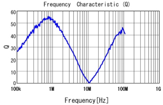
■ LQH3NPZ101MME Q
