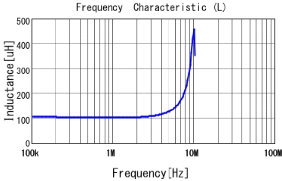
■ LQH3NPZ101MME L
