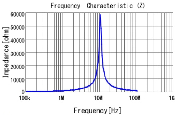
■ LQH3NPZ101MME |Z|
