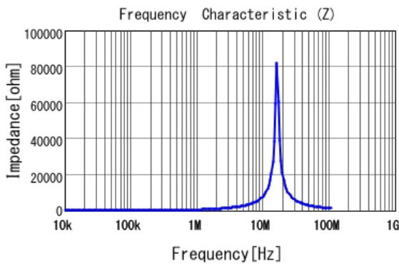
■ LQH2MPN820MGR |Z|
