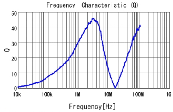
■ LQH2MPN820MGR Q
