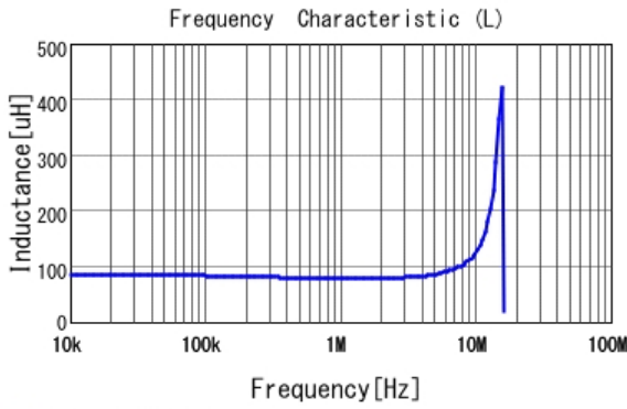
■ LQH2MPN820MGR L
