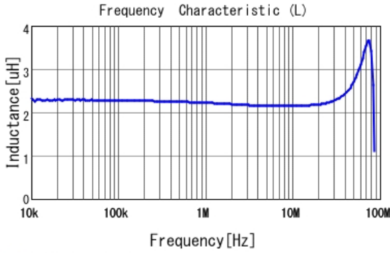
■ LQH2HPN2R2MJR L
