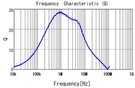
■ LQH2HPN2R2MJR Q
