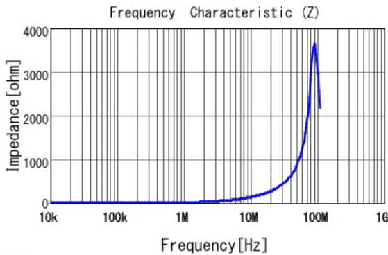
■ LQH2HPN2R2MJR |Z|
