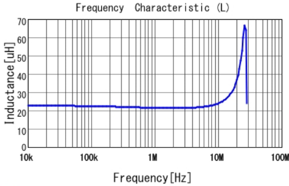
LQH2HPN220MJR L
