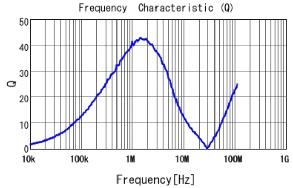
LQH2HPN220MJR Q
