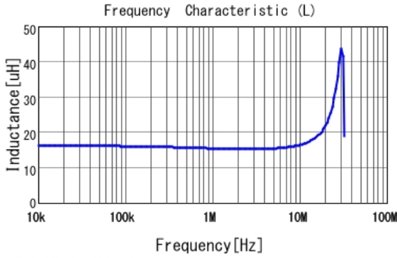
■ LQH2HPN150MJR L
