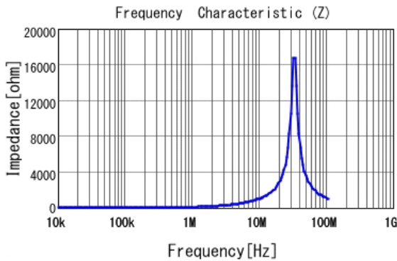
■ LQH2HPN150MJR |Z|
