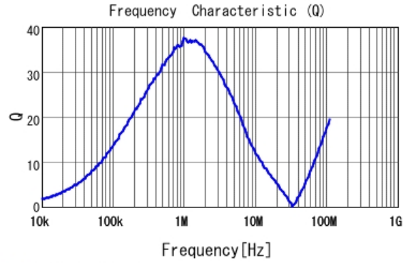
■ LQH2HPN150MJR Q
