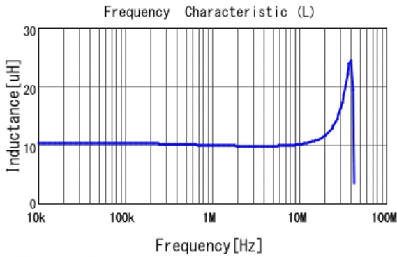
■ LQH2HPN100MJR L
