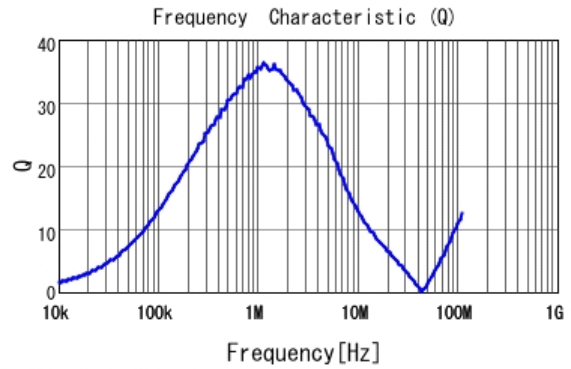
■ LQH2HPN100MJR Q
