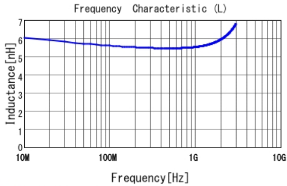
■ LQG15WZ5N6C02 L
