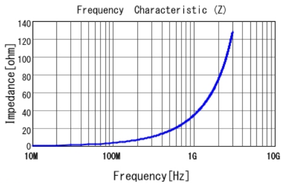
■ LQG15WZ5N6C02 |Z|
