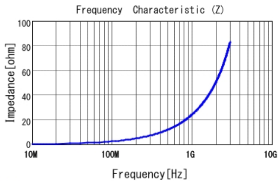
■ LQG15WZ3N9S02 |Z|
