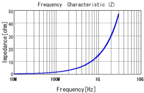
■ LQG15WZ2N4B02 |Z|
