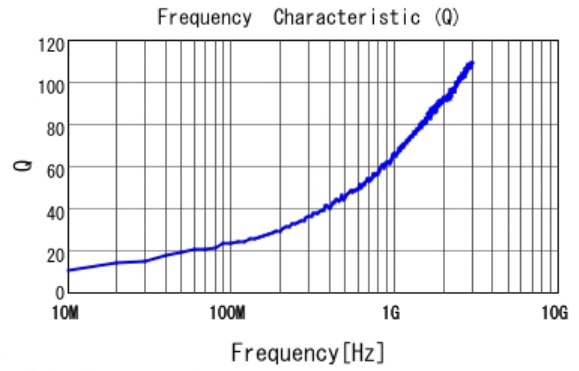
■ LQG15WZ1N5B02 Q
