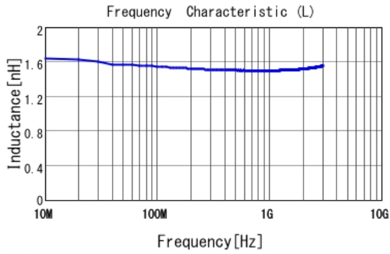
■ LQG15WZ1N5B02 L
