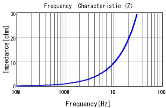
■ LQG15WZ1N5B02 |Z|
