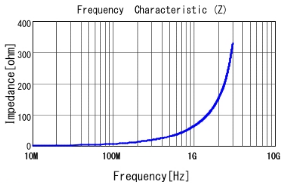
■ LQG15WZ10NH02 |Z|
