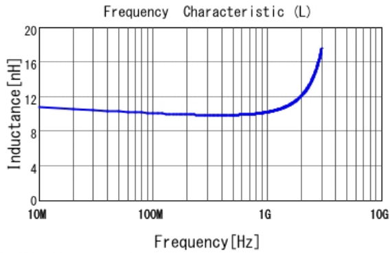
■ LQG15WZ10NH02 L
