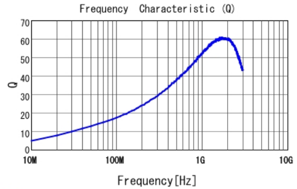
■ LQG15WZ10NH02 Q
