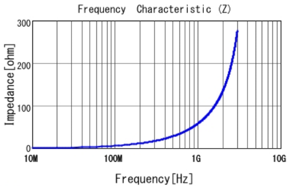
■ LQG15WH9N1J02 |Z|
