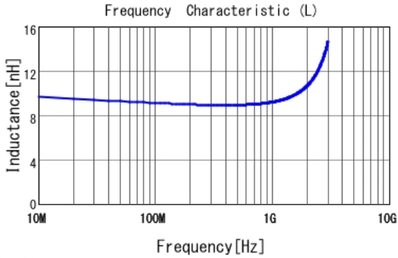
■ LQG15WH9N1J02 L
