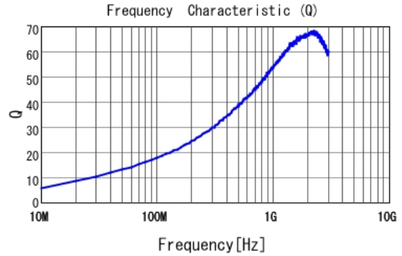
■ LQG15WH7N5G02 Q
