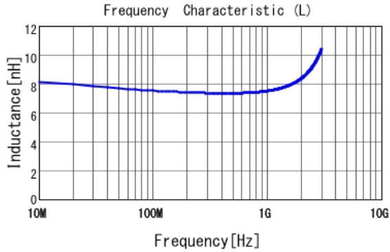
■ LQG15WH7N5G02 L
