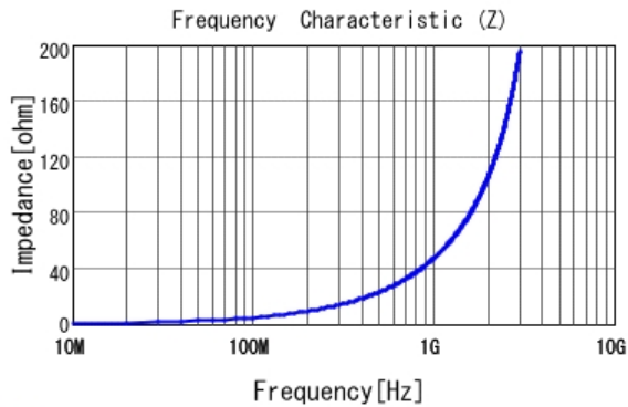
■ LQG15WH7N5G02 |Z|
